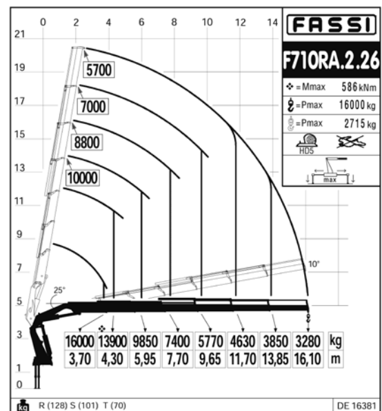
Traglast 710 ohne Jip
