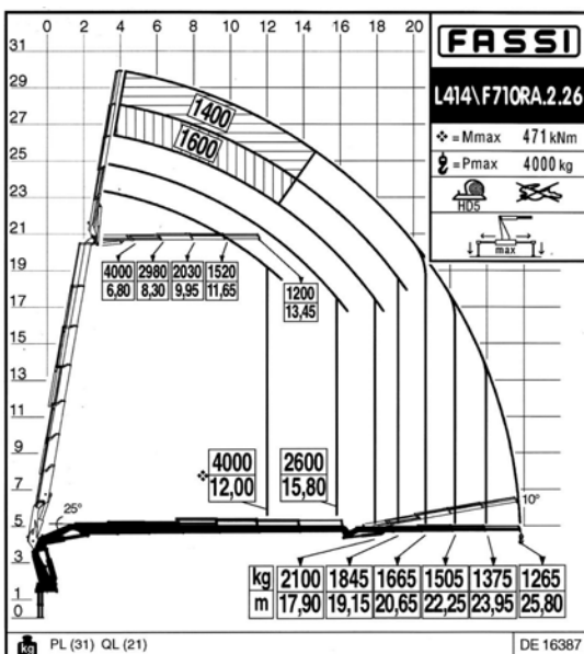
Traglast 710 mit Jip
